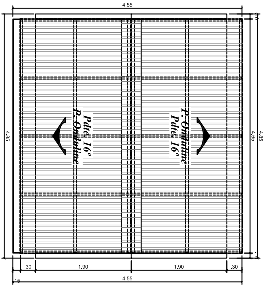
TECHOS Escala: 1-50
